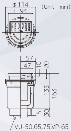
HSKT type
